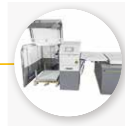
柯达超胜Q800直接制版机， 搭载多托盘上版机
