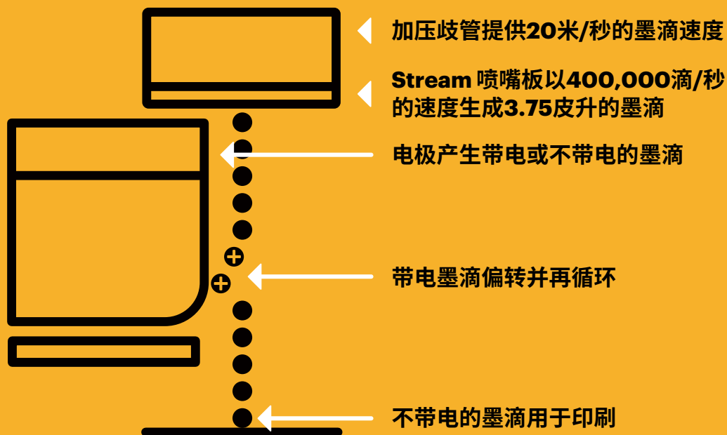
图2: 静电墨滴选择
