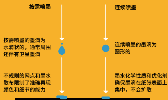
图4: 墨滴形状比较
